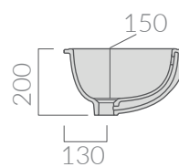
Sezione Section
