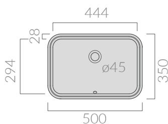
Vista dall'alto Top View
