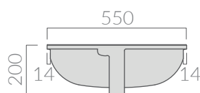
Vista parte frontale Frontal View
